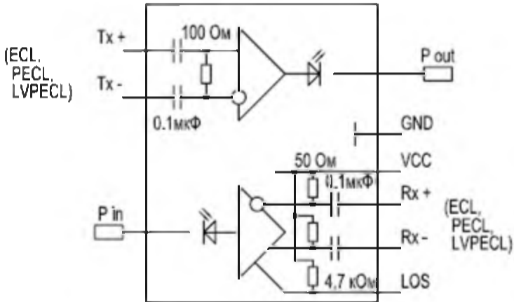
Рисунок 1 - Упрощённая схема модуля
