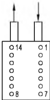
Рисунок 2 - Назначение выводов
