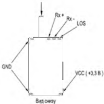
Рисунок 2 - Назначение выводов
