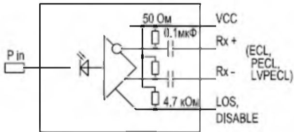
Рисунок 1 - Упрощённая схема модуля
