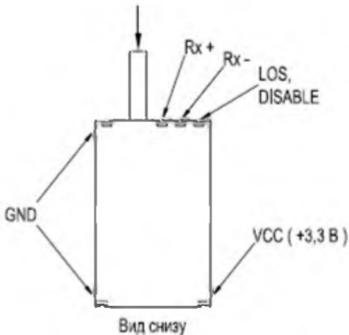
Рисунок 2 - Назначение выводов
