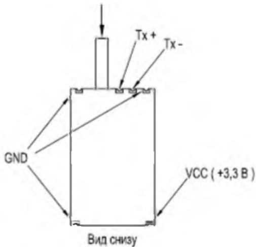
Рисунок 2 - Назначение выводов
