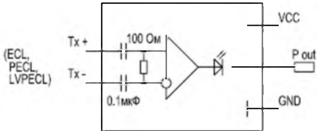
Рисунок 1 - Упрощённая схема модуля
