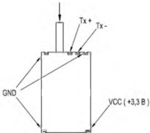
Рисунок 2 - Назначение выводов
