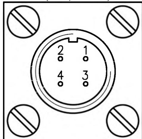
Вилка РСГ4ТВ (XP2, «27 В»)
