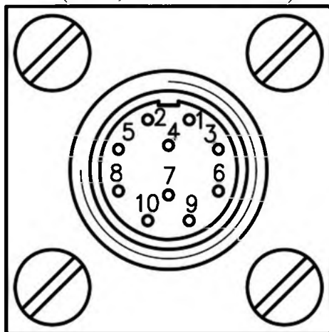
Вилка MP1-10-2-B (XP1, «1000Base-T»)
