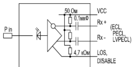
Рисунок 1 - Упрощённая схема модуля
